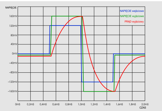
Symulacja pracy wzmacniacza napięciowego
